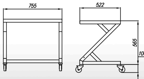
СХЕМА ПОДСТАВКИ
